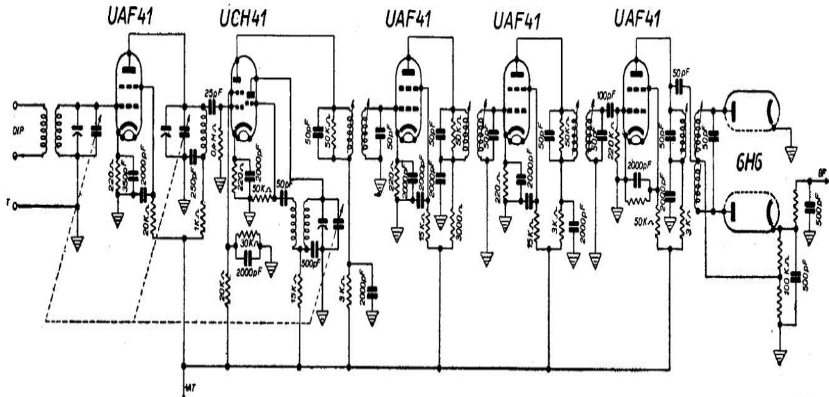
ASTARS (F.lli Nicola) - Mod. RG/2 - Adattatore a modulazione di frequenza, gamma da 88 a 108 megacicli. Sensibilità da 2 a 5 micro-volt. Alimentatore anodico eventuale a parte.
